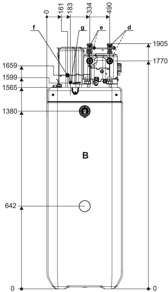
300 Litres Dimensions side-view
