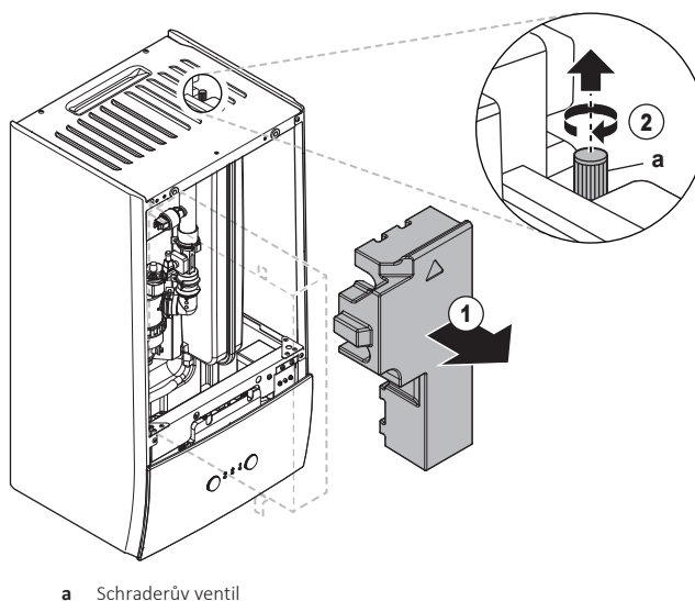
a Schraderův ventil
