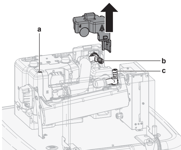
a, b, c Ruční odvzdušňovací ventil
