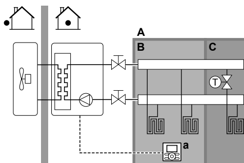
A Hlavní zóna teploty výstupní vody B Místnost 1 C Místnost 2 a Uživatelské rozhraní
