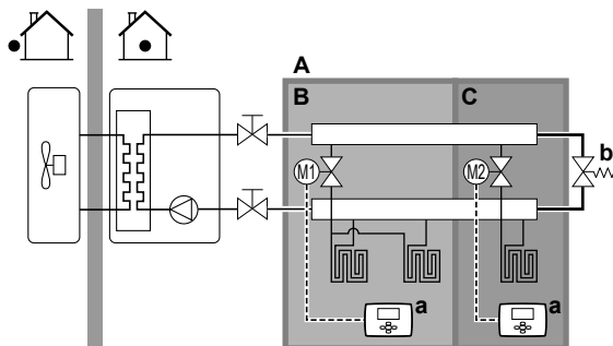
A Hlavní zóna teploty výstupní vody B Místnost 1 C Místnost 2 a Externí pokojový termostat b Obtokový ventil
