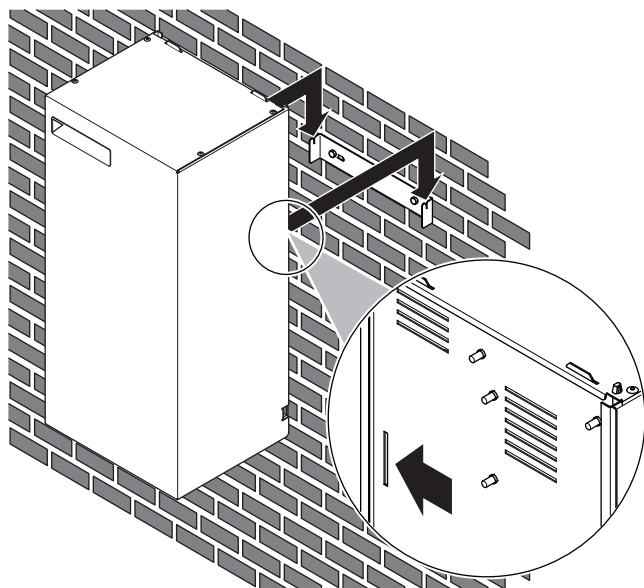
2 Zavěste záložní ohřívač na nástěnný držák.
