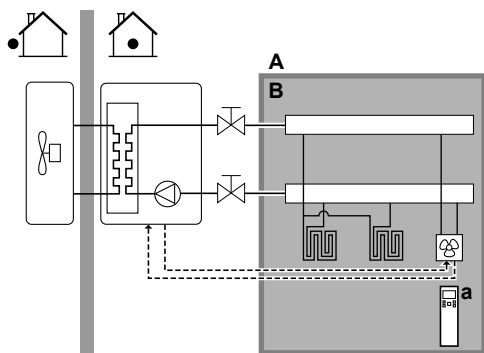
A Hlavní zóna teploty výstupní vody B Jedna samostatná místnost a Dálkový ovladač konvektorů tepelného čerpadla
