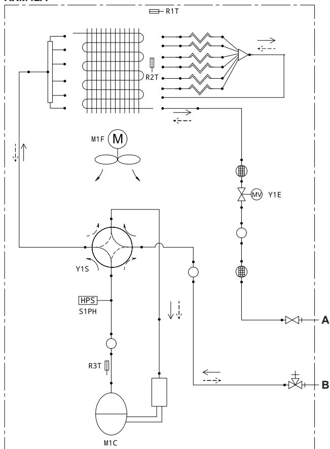
Legenda schématu potrubí
