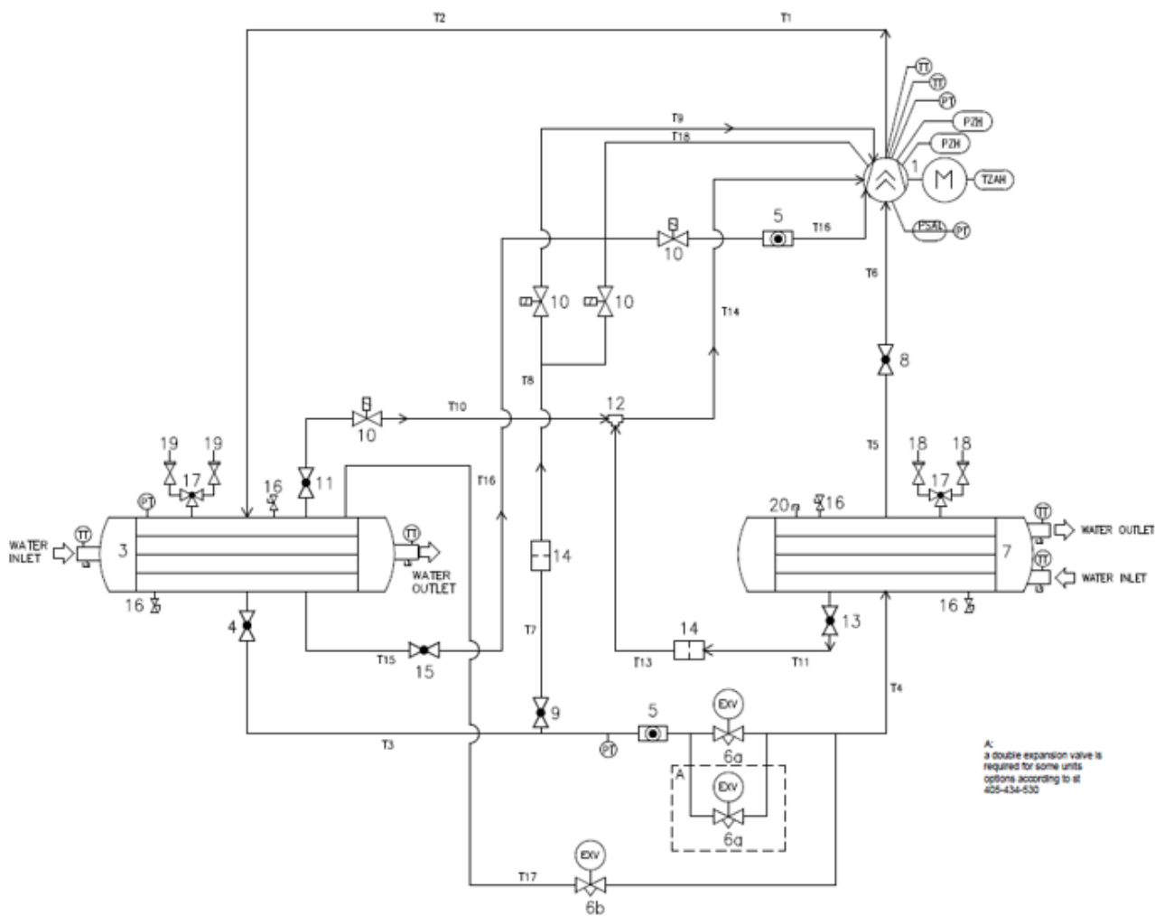
Obrázek14 - P&ID Možnost.251
