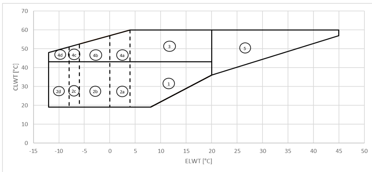
Obrázek10 – EWWS_VZ_SS
