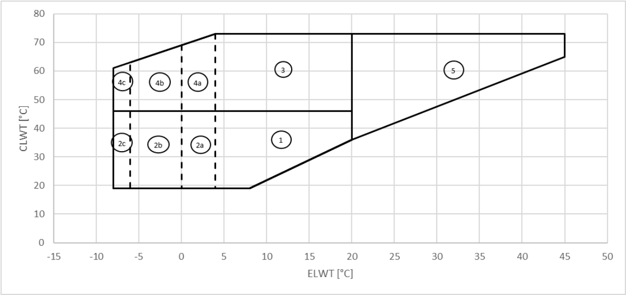
Obrázek7 – EWWH_VZ_SS
