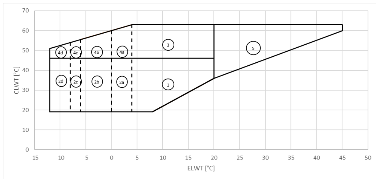
Obrázek5 – Pouzdro EWWD_VZ_SS
