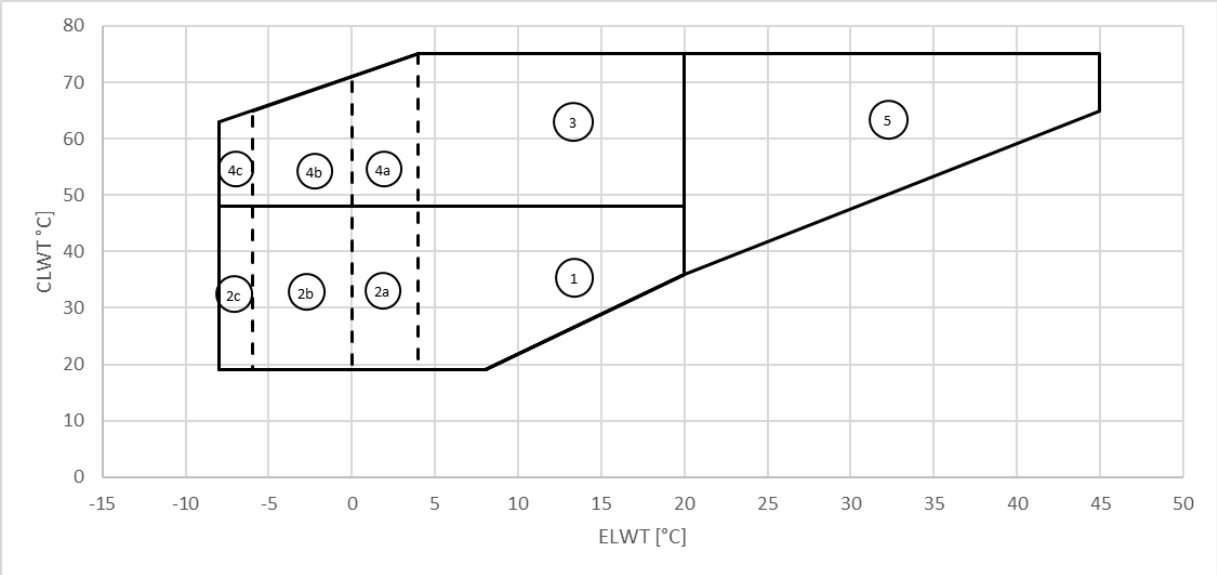
Obrázek8 – EWWH_VZ_XS
