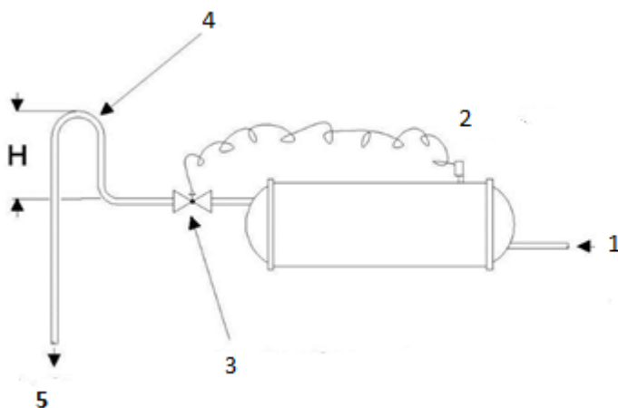
Obrázek13 – Systém řízení kondenzace podpovrchovou vodou
