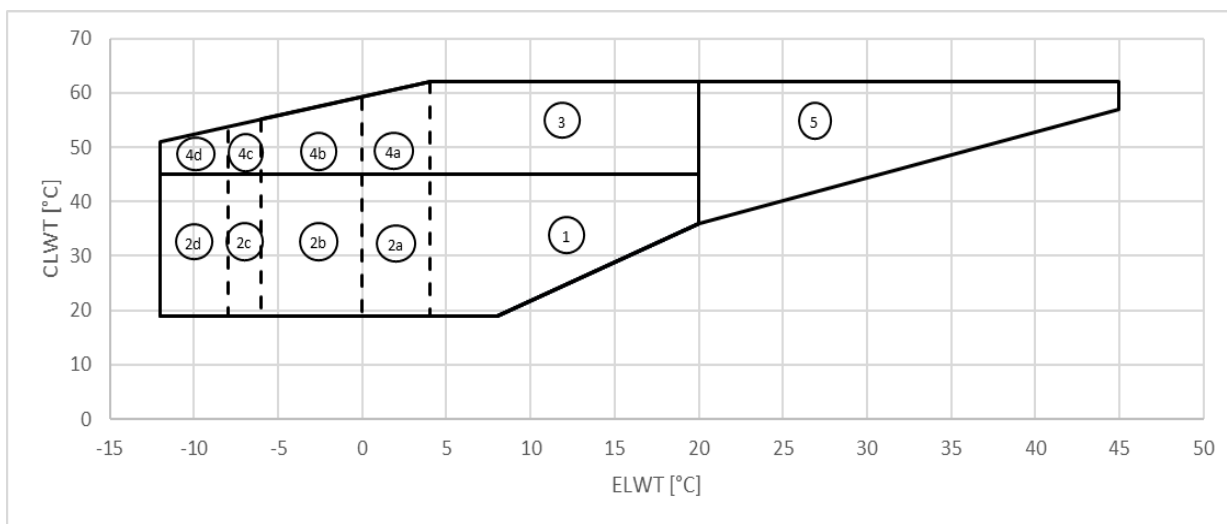
Obrázek11 –EWWS_VZ_XS/PS
