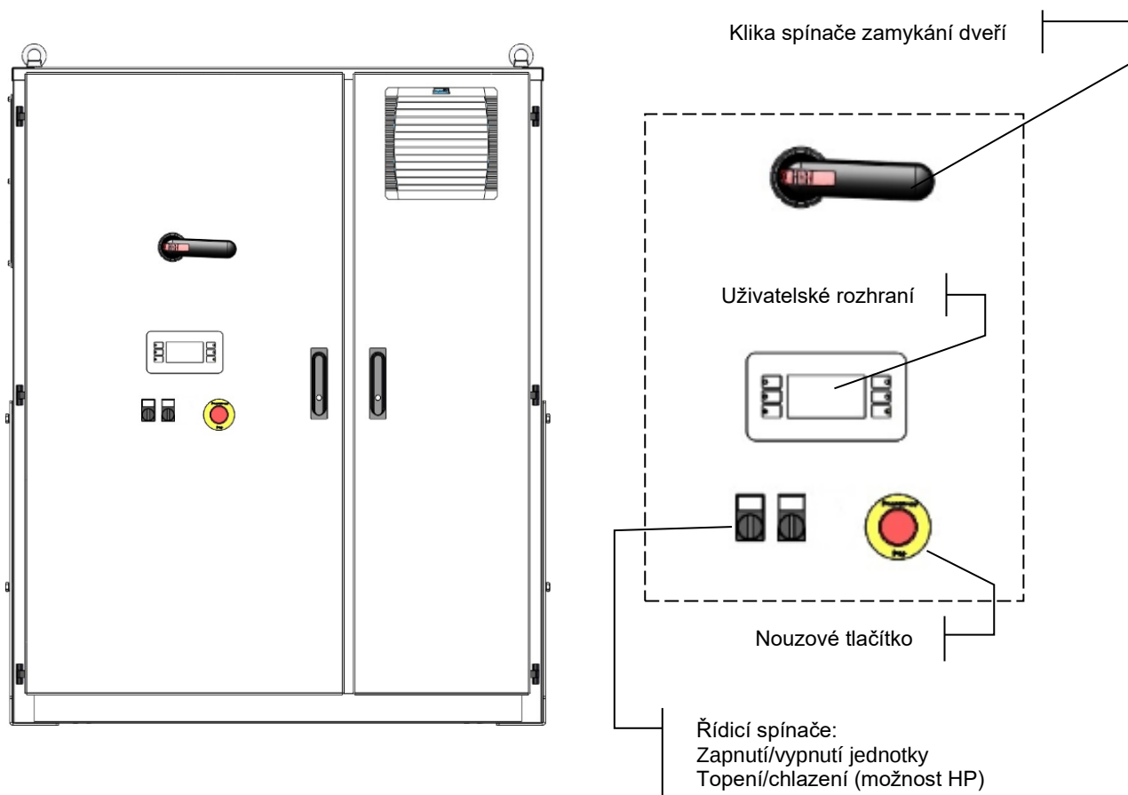
Obrázek15 – Rozhraní jednotky
