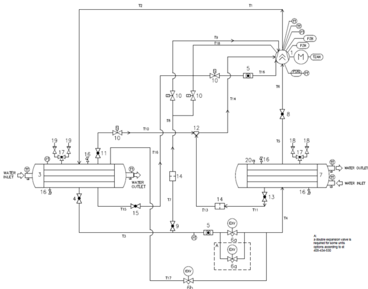
Obrázek14 - P&ID Možnost.251
