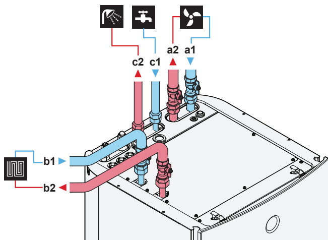
a1 Doplňková zóna – Prostorové vytápění/chlazení – VSTUP vody (šroubová přípojka, 1")
