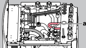
a Potrubí chladiva v plynném stavu
