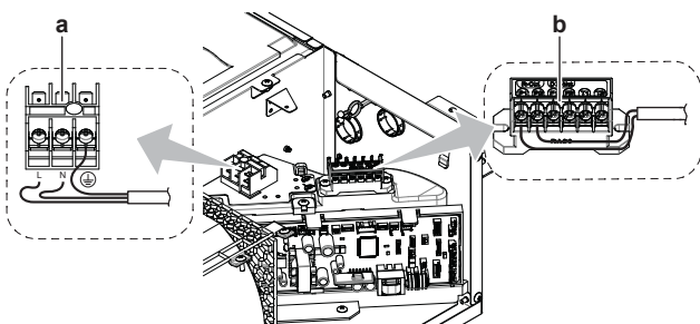
a Svorkovnice napájení b Svorkovnice uživatelského ovladače
