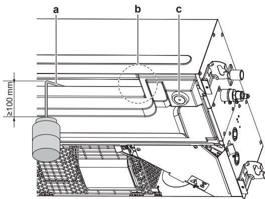
a Plastový zásobník na vodu o délce trubky \geq 100 mm b Umístění vypouštěcího čerpadla a plovákového spínače c Výpust' odpadní vody (s pryžovou zátkou). Tato výpust' odpadní vody se používá k vypuštění vody z vypouštěcí vany.
