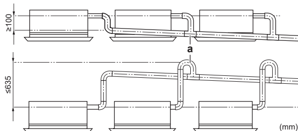
a Rozdvójka (spojka T)
