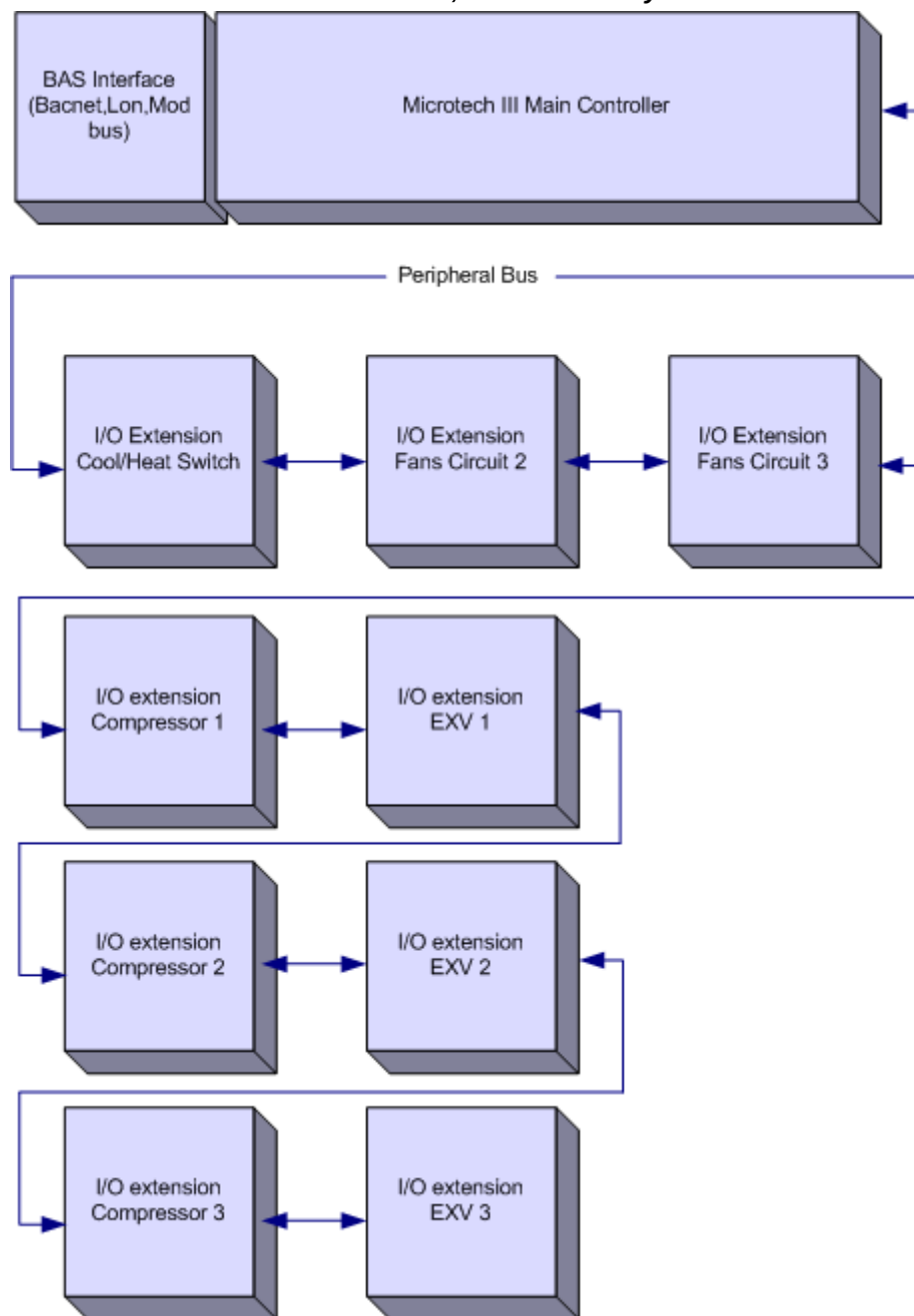
Obrázek 4, Architektura systému
