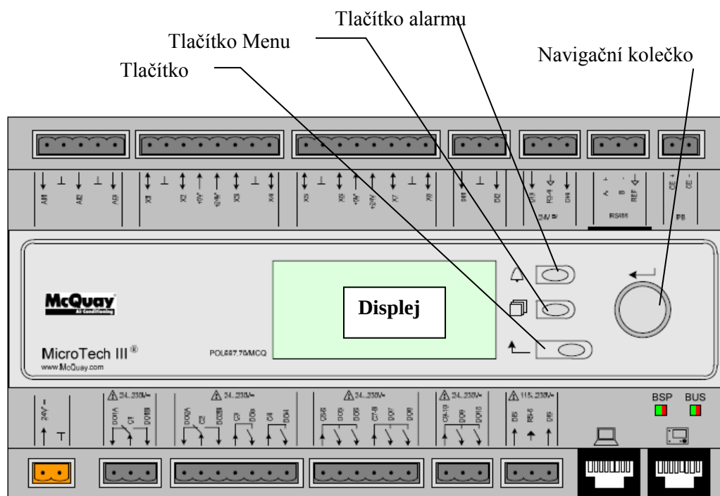
Obrázek 7, řídicí jednotka
