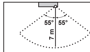
Vodorovný úhel (pohled shora)
