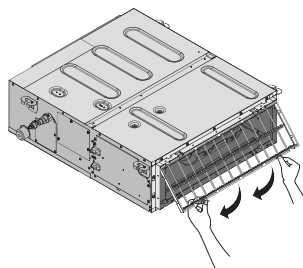
nasávání zadem
