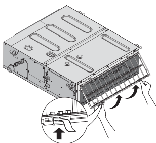
nasávání zadem
